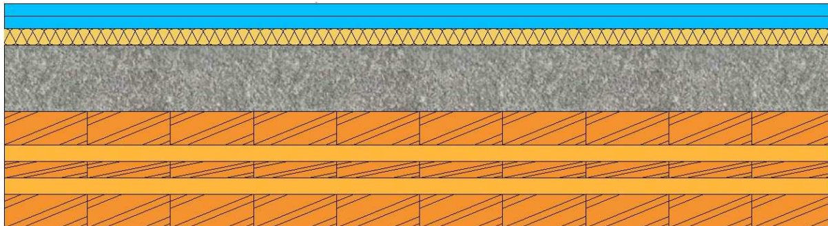
Abbildung 1: Vertikalschnitt BHB 1.10 20 mm MiWo, TRI
